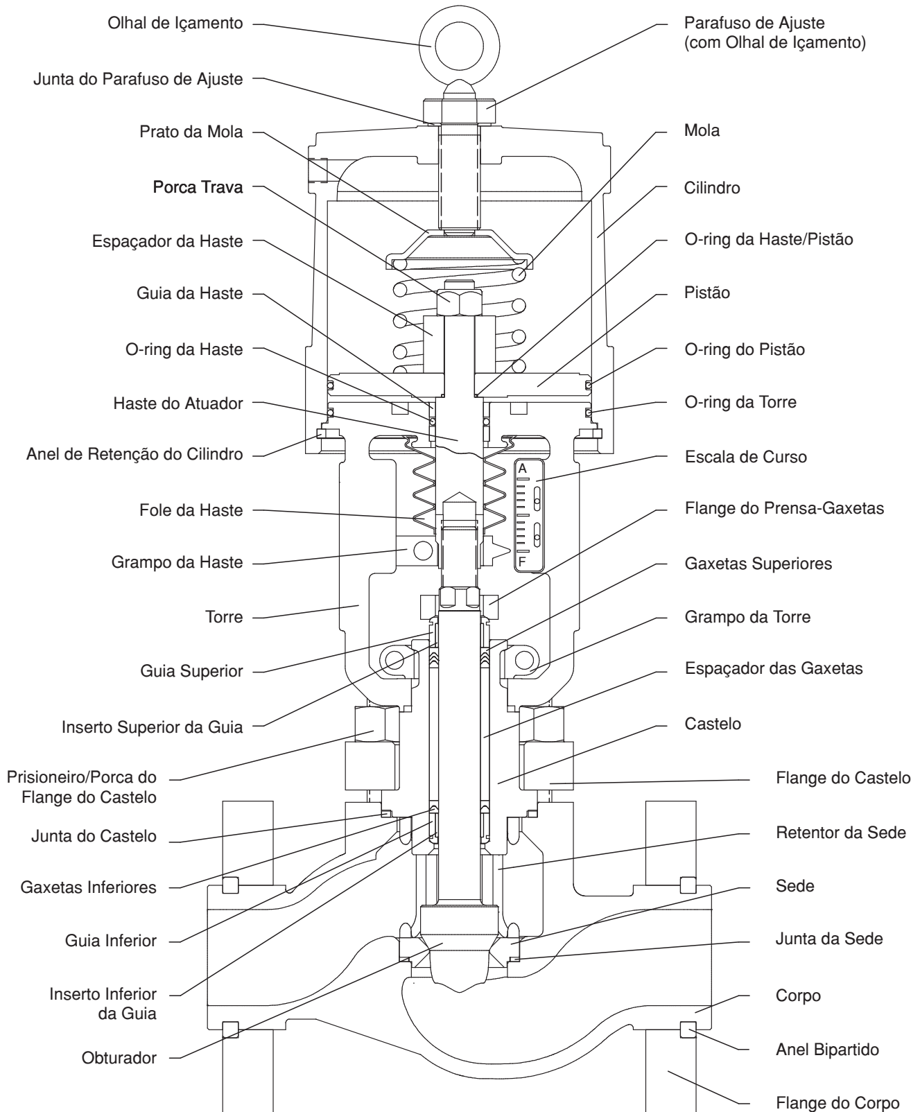
Figura 2 - Válvula de controle GL5
